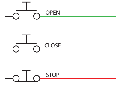
Wiring Schematic
